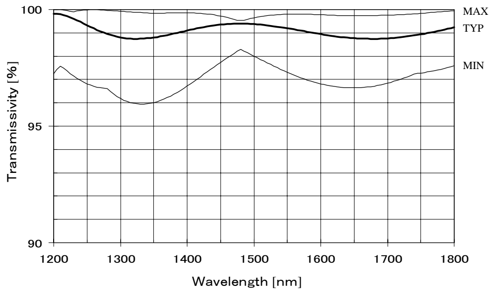
分光両面透過率チャート
