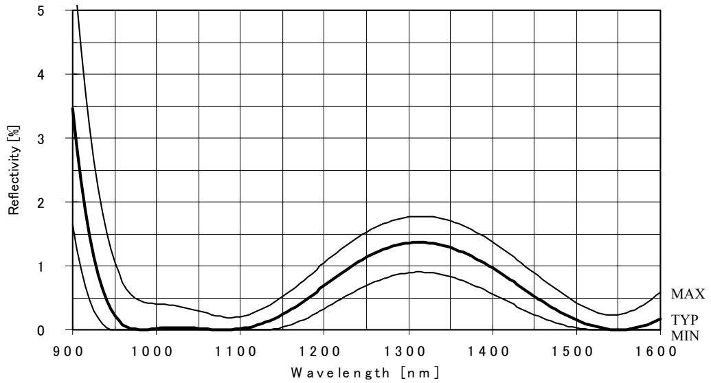
分光片面反射率チャート
