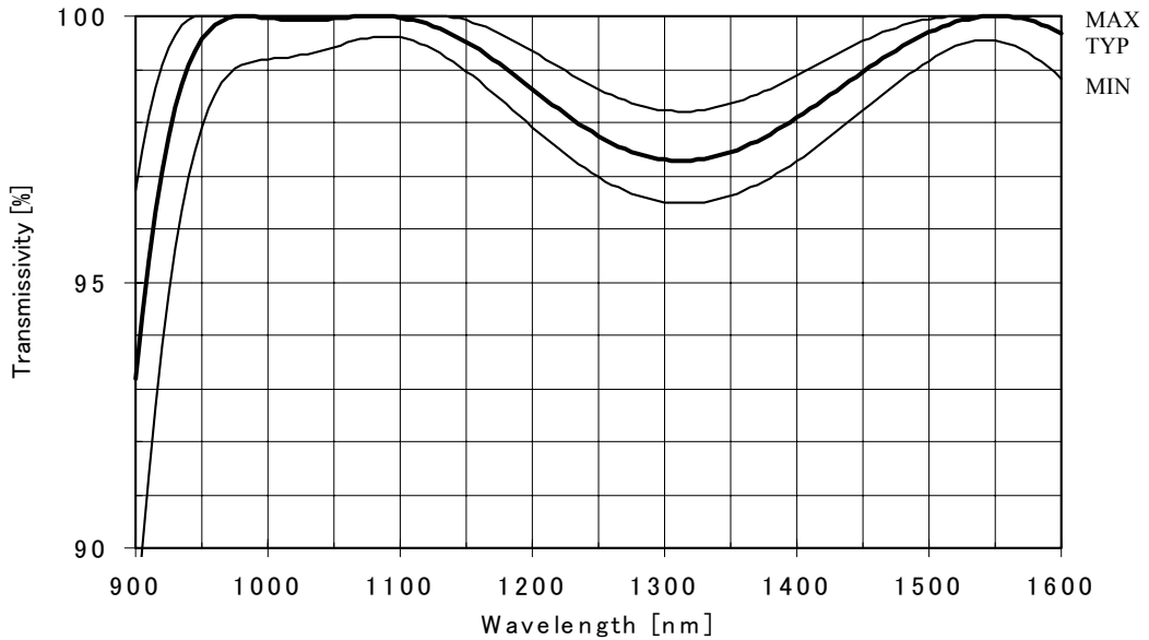
分光両面透過率チャート
